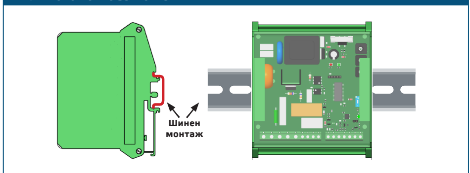
Фиг. 2 Положение за монтаж
