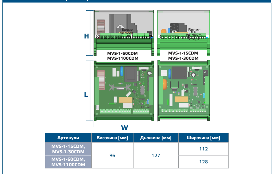
Фиг. 1 Монтажни размери
