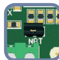
Фиг. 5 Джъмпер за съгласуващия резистор
