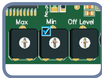
Фиг. 7 Тример за настройка на мин. обороти
