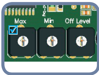
Фиг. 6 Тример за настройка на макс. обороти
