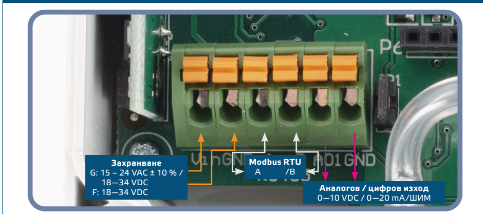
Фиг. 3 Свързване
