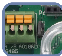
Фиг. 5 Свързан джъмпер за съгласуващия резистор
