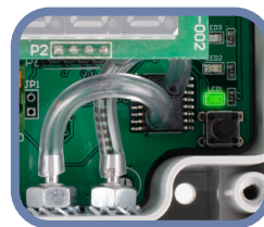
Фиг. 7 Индикация за захранване / комуникация по Modbus
