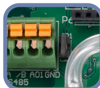
Фиг. 5 Джъмпер за съгласувания резистор 1
