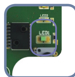
Фиг. 5 Индикация за захранване /Modbus комуникация
