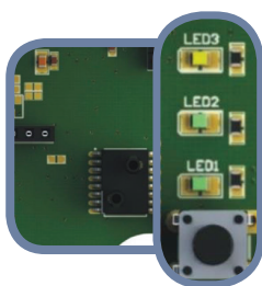
Фиг. 6 Бутон за стартиране на процедури за калибриране на датчика и възстановяване на фабричните Modbus настройки
