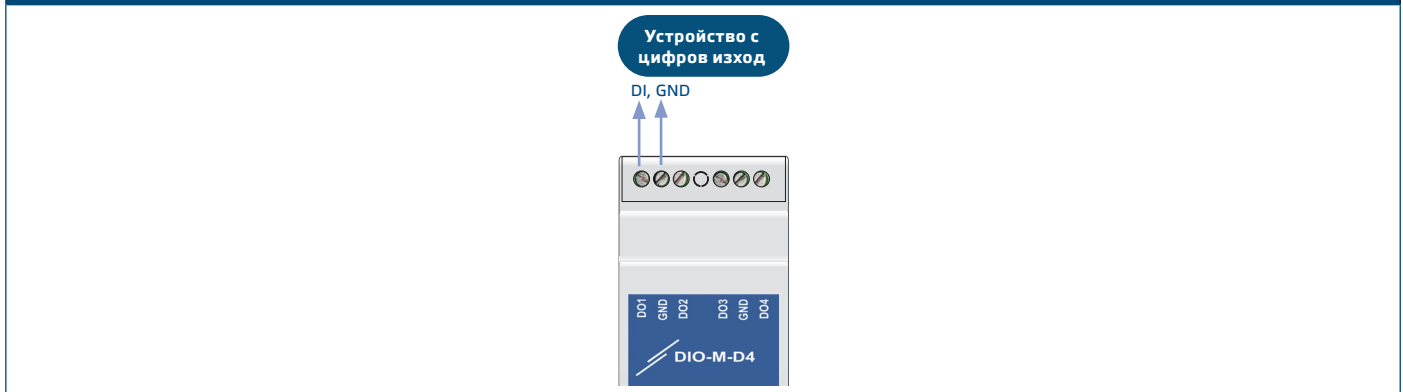
Фиг. 5 Типични примери за свързване - цифрови изходи
