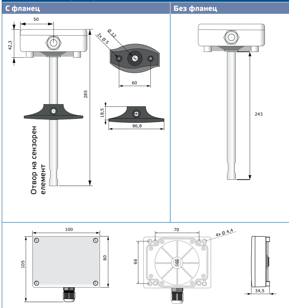
Фиг. 1 Монтажни размери
