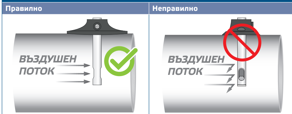
Фиг. 2 Положение за монтаж
