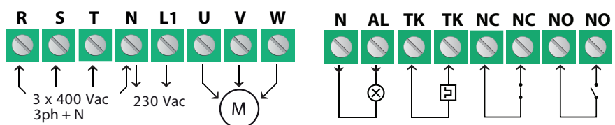
Фиг. 3 Електрическа схема
