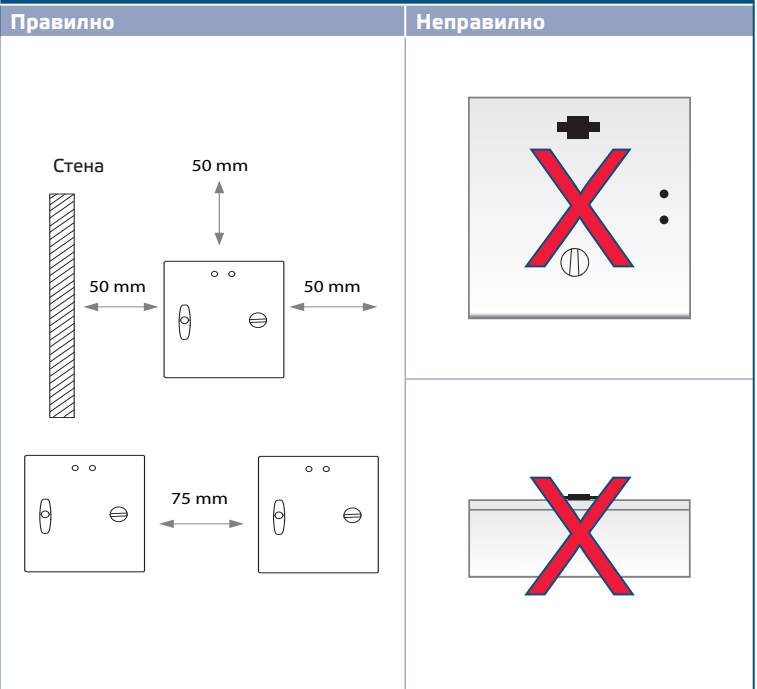
Фиг. 2 Положение за монтаж
